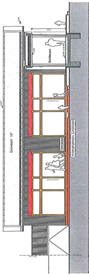
ANSICHT NORD
